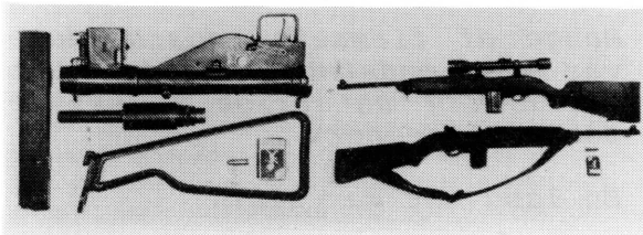
Sten-Gun maskinpistol. Magasinet til venstre indeholder 30 patroner. US-carabin med og uden kikkertsigte. Magasinet indeholder 14 patroner.
